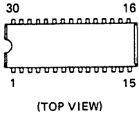
LA1851N
